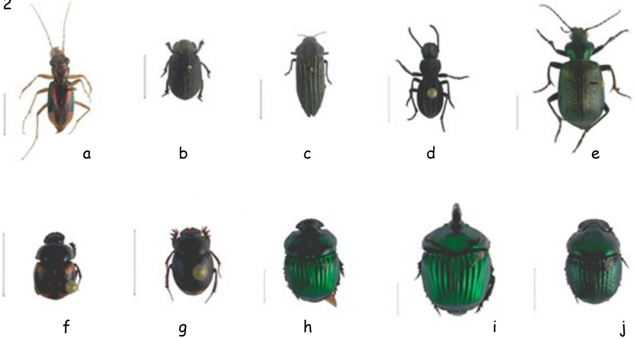
Fig. 2.- Algunos coleópteros del sector "La Greda". a.- Tetracha carolina . b.- Omorgus suberosus . c.- Polycesta bicolor . d.- Psammeticus sp. e.- Calosoma abbreviatum . f.- Canthon baltheatus . g.- Canthon fuscipes . h.- Phanaeus lunaris (hembra). i.- Phanaeus lunaris (macho). j.- Phanaeus sp. La escala equivale a 1 cm. (Fotografías tomadas por los autores).
